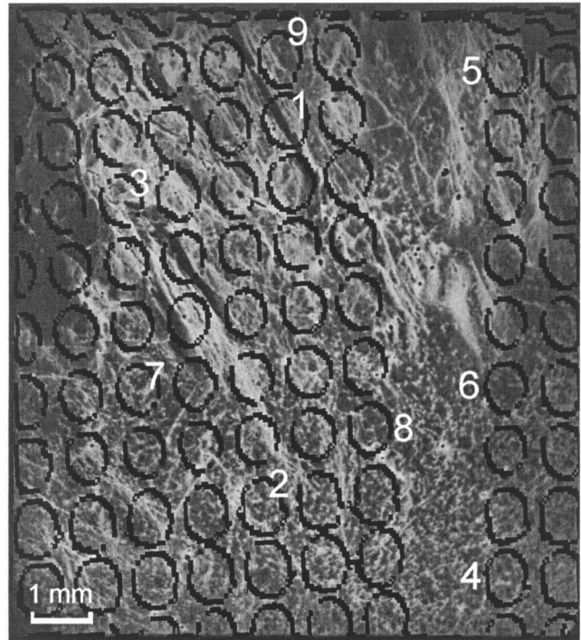
Рис. 2. Карта расположения диодов Шоттки, спроецированная на рентгенографическое изображение. Окружности обозначают места нахождения диодов Шоттки на пластине. Номера диодов Шоттки на карте соответствуют номерам в табл. 2.
