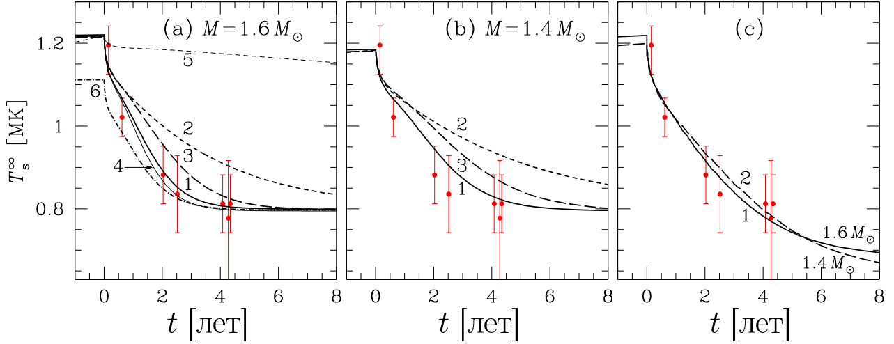
Рис. 4. Теоретические кривые остывания нейтронных звёзд массой (a) M = 1.6M_{\odot} и (b) M = 1.4M_{\odot} , и (c) звёзд обеих масс в сравнении с наблюдениями рентгеновского транзиента KS 1731–260. Время t отсчитывается от момента окончания аккреции. Кривые описаны в таблице 1 и в тексте.
