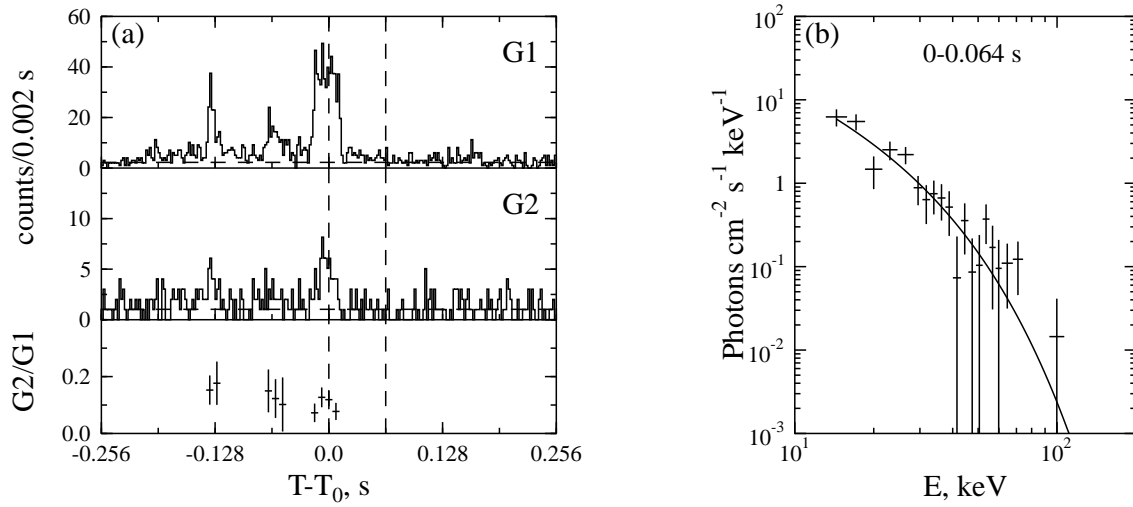
Fig. 5.8.— Burst 980618f.
