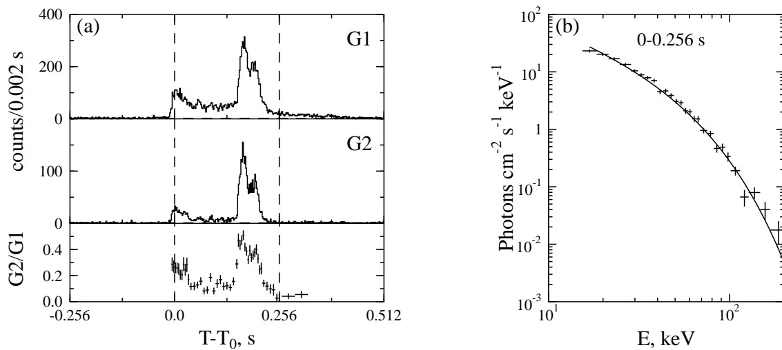
Fig. 5.10.— Burst 980618h.
