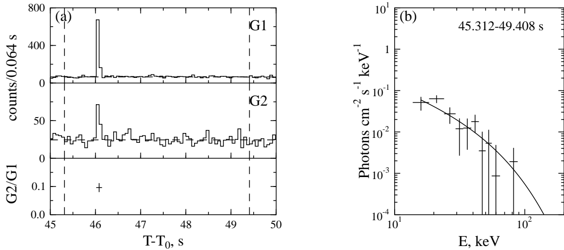
Fig. 4.4.— Burst 961118b (continued).
