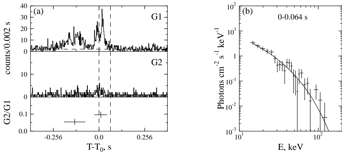
Fig. 4.6.— Burst 961119a (Kosmos 2326).
