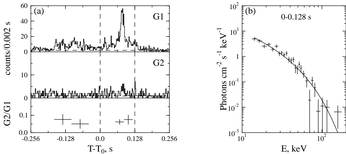
Fig. 4.5.— Burst 961118d (Kosmos 2326).
