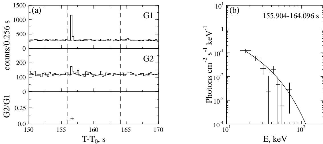
Fig. 3.52.— Burst 981013a (continued).
