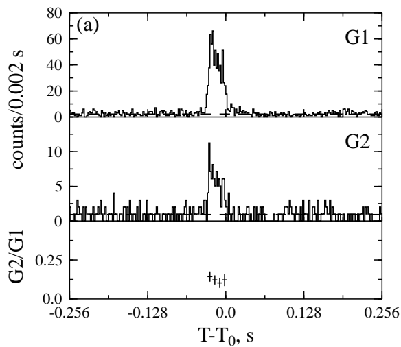
Fig. 3.47.— Burst 980912.
