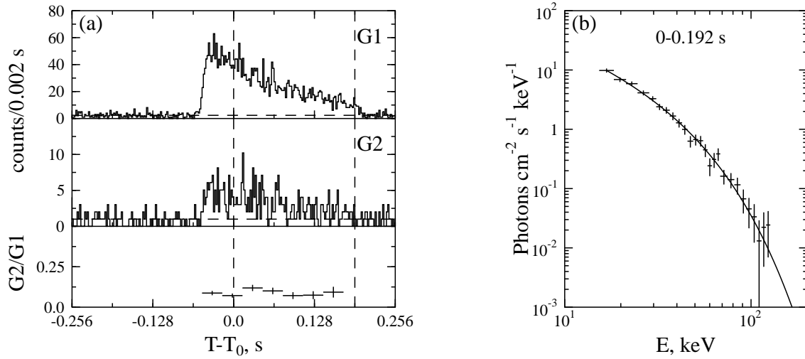
Fig. 3.45.— Burst 980902b.
