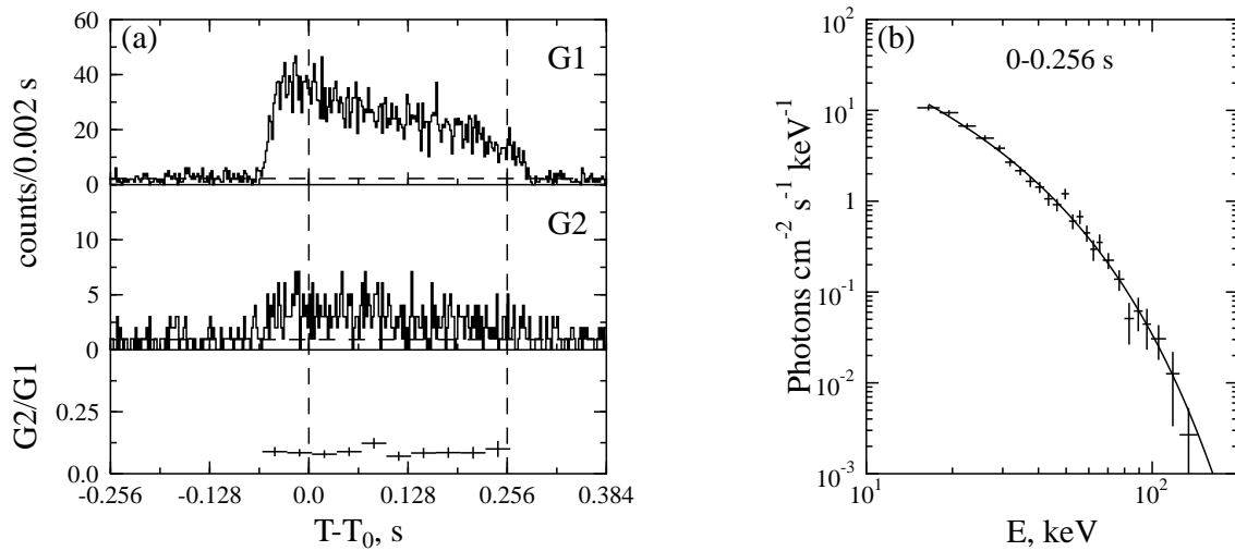
Fig. 3.46.— Burst 980911.
