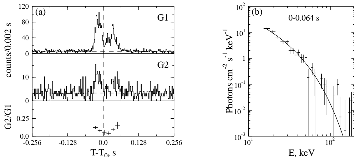
Fig. 3.33.— Burst 980828.
