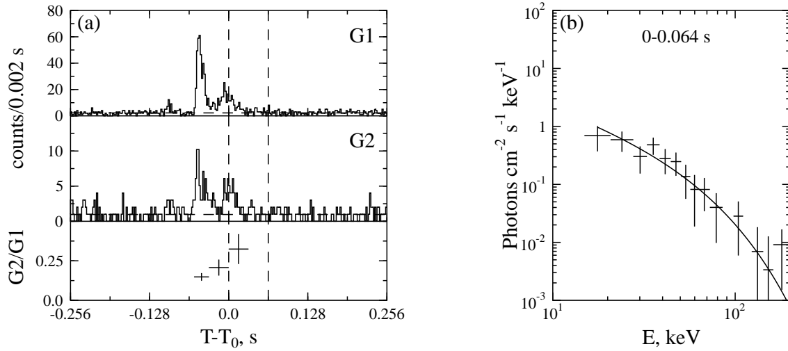
Fig. 3.20.— Burst 980607b.
