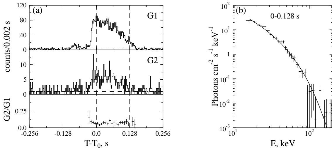
Fig. 3.21.— Burst 980616a.
