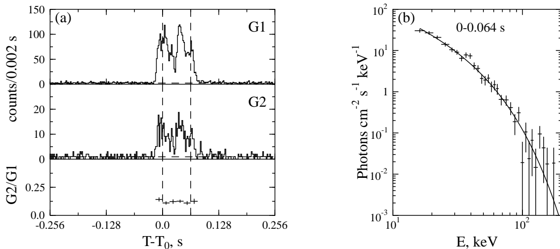
Fig. 3.22.— Burst 980616b.
